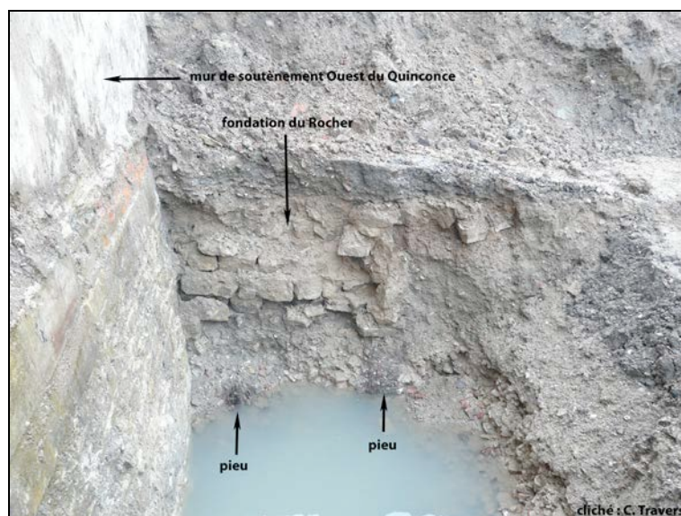
fig. 66 : Vestiges de la fondation du Rocher – Coupe E-0 du sondage S.XXI
