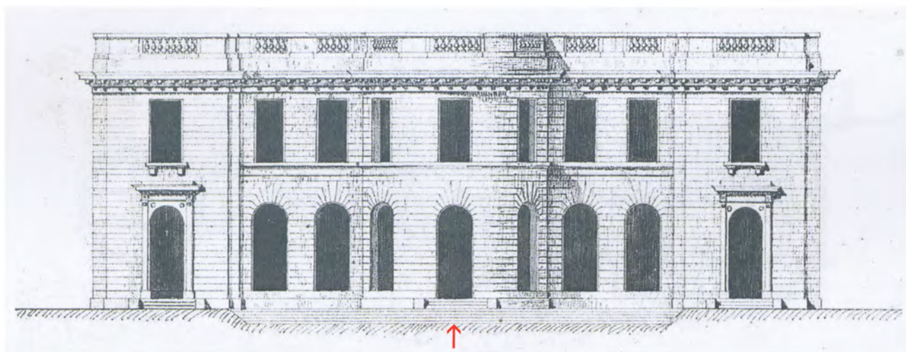
A.-T. Brongniart, Hôtel Bourbon-Condé, rue Monsieur : corps de logis entre cour et jardin, élévation sur jardin , 1780 Bibliothèque nationale, Département des estampes et de la photographie, Collection Destailleur, Rés Ve-53 (j) (cliché BNF)
