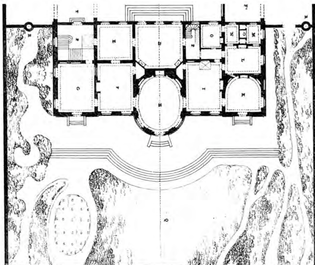
J.-C. Krafft, N. Ransonnette, Maison de M lle de Condé, vue sur le boulevard Plumet, bâtie par Brongniart, architecte, s. d. (avant 1801), détail Extrait de : J.-C. Krafft, dessinateur, et N. Ransonnette, graveur, Plans, coupes élévation des plus belles maisons et des hôtels construits à Paris et dans les environs, Paris, 1801, planche 61 (cliché GRAHAL)
