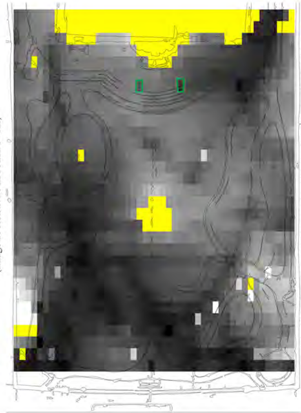
ill. 62a : Anomalie liée à la présence d'un élément maçonné XVIII e (Image de résistivité EPICEHA - 1m)
