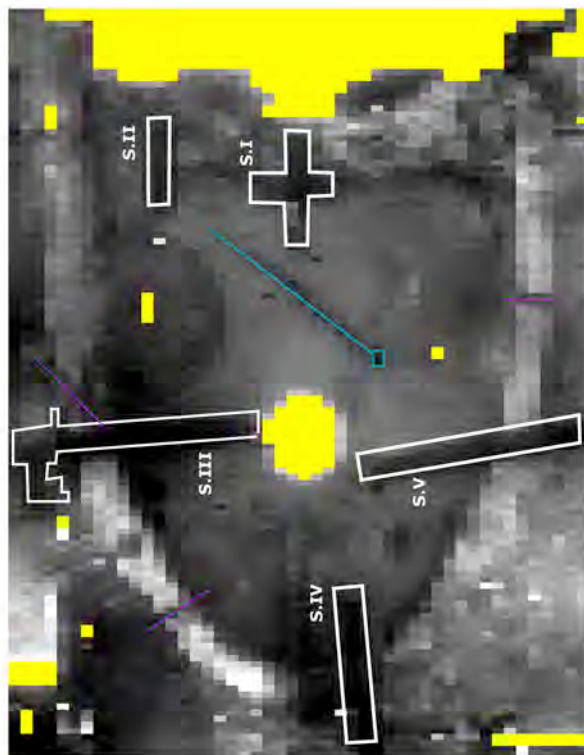
ill. 61a : Anomalies liées à des structures XXè et contemporaines (Image de résistivité EPICEHA - 0,5m)
