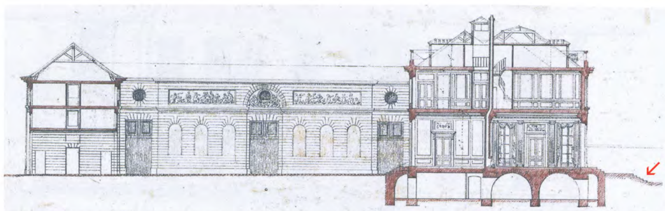
A.-T. Brongniart, Corps de logis sur rue et corps de logis entre cour et jardin : coupes et corps de logis en aile à gauche : élévation sur cour ; jointes au devis et marché pour la construction d'un hôtel du 19 juin 1780. Château de Chantilly, Bibliothèque, Cabinet des titres, Hôtels et maisons de la maison de Condé, 1-AC-015 (cliché GRAHAL)
