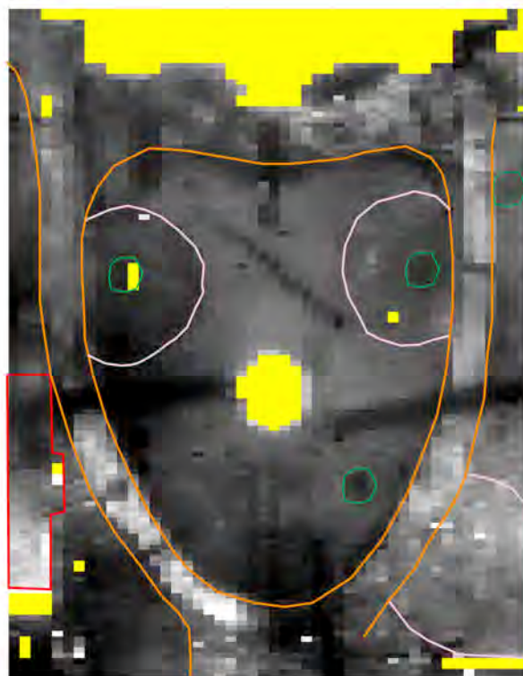
ill. 61b : Anomalies liées aux aménagements de la fin du XIXè (Image de résistivité EPICEHA - 0,5m)
