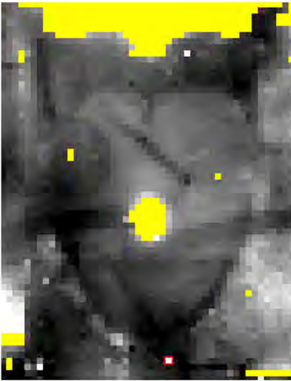
ill. 62a : Anomalie liée à la présence d'un élément maçonné XVIII e (Image de résistivité EPICEHA - 1m)
