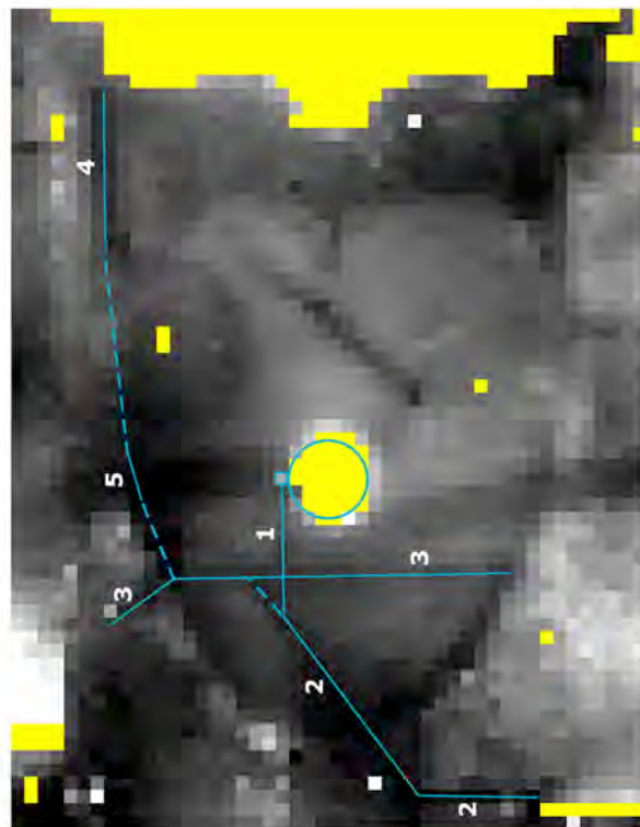
ill. 61c : Anomalies liées aux structures hydrauliques de la fin du XIXè (Image de résistivité EPICEHA - 1m)
